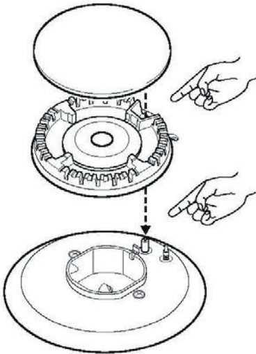
Partes del quemador
